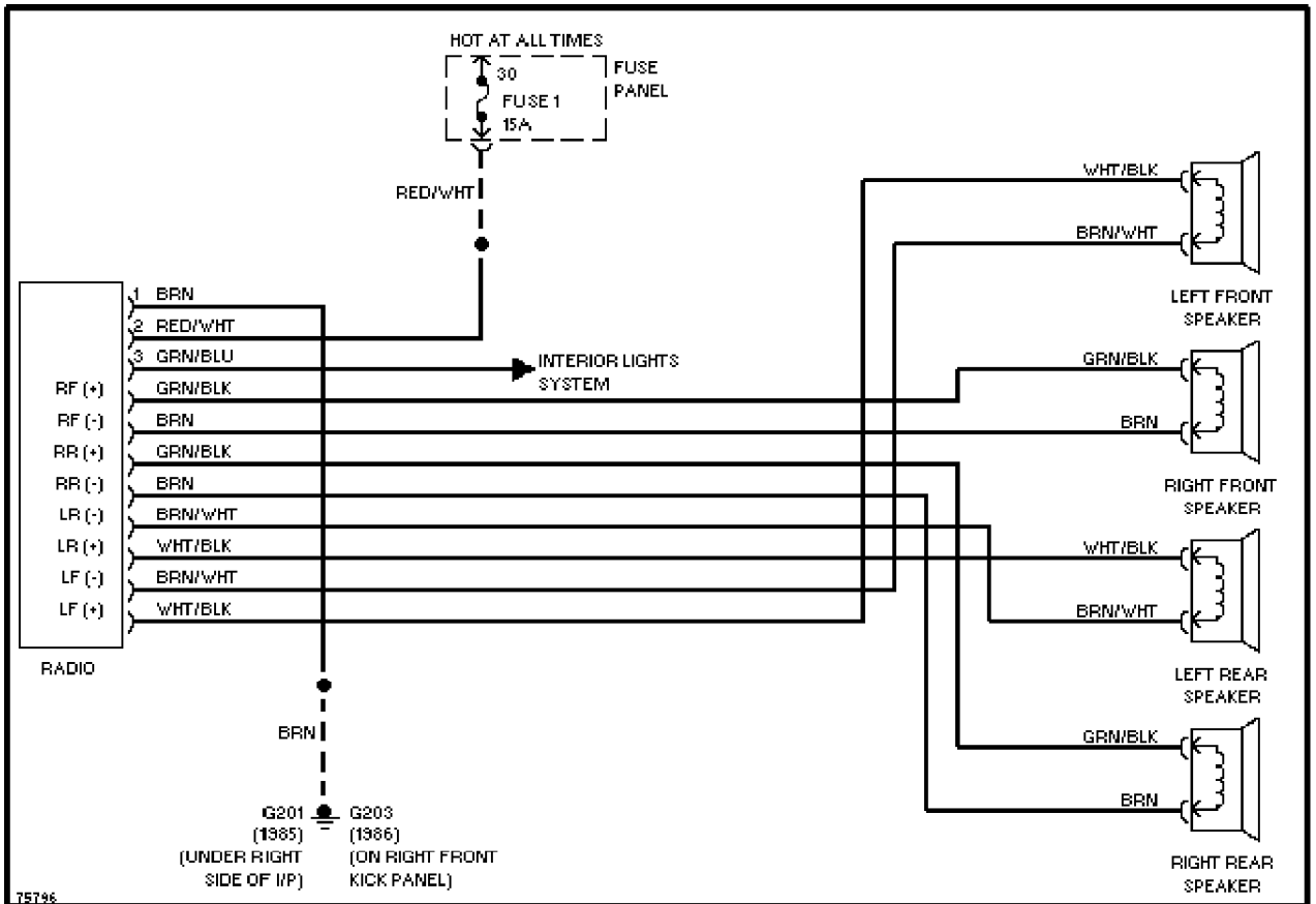
Radio Circuits
