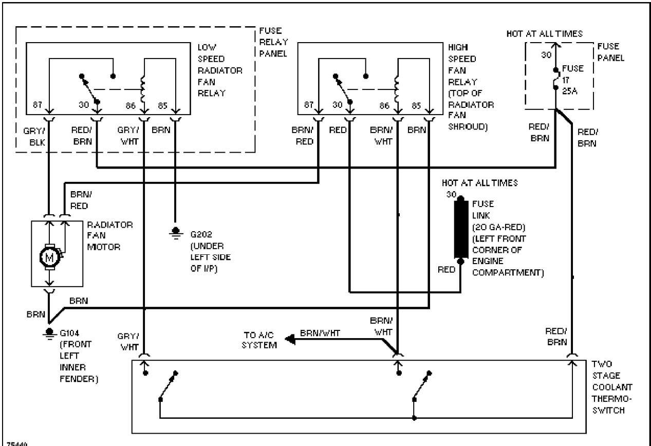
75440 Cooling Fan Circuit
